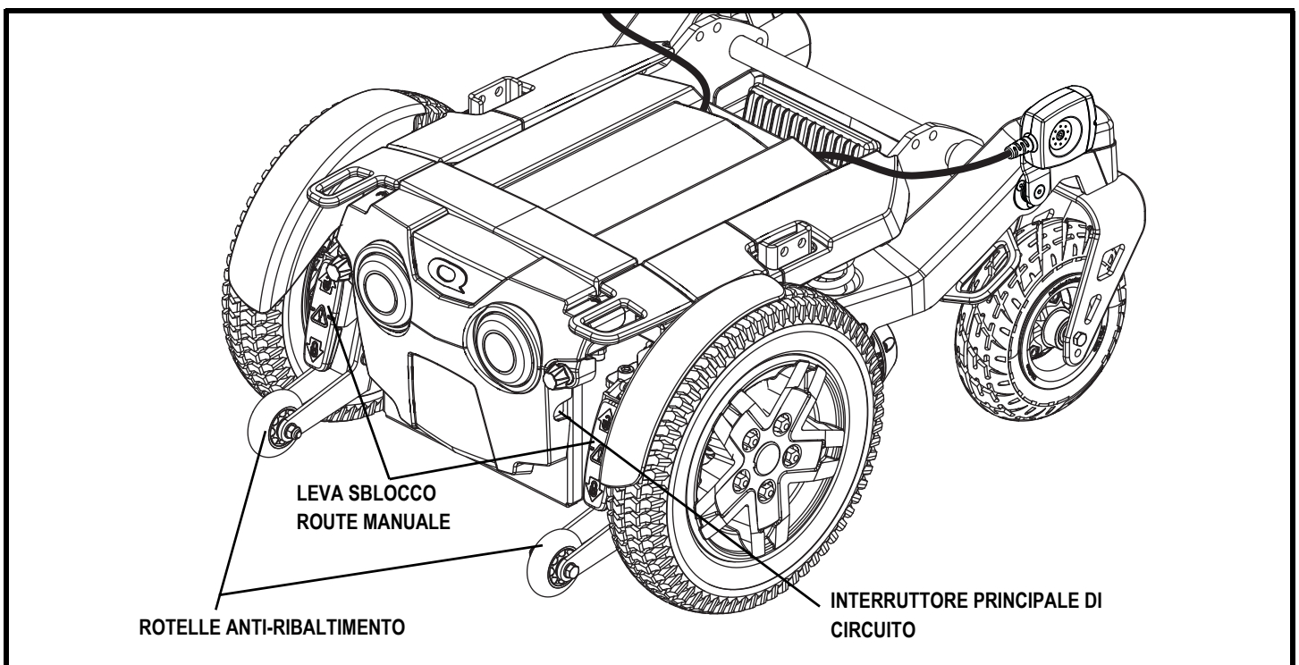
Figura 6. La base di alimentazione della R44
