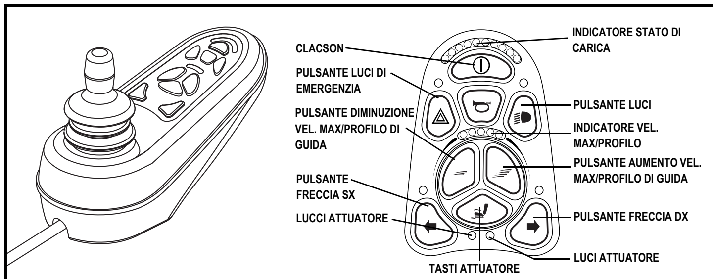
Figura 13. Centralina e Tastiera
