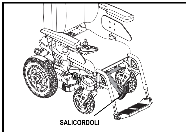
Figura 7. La R44 con il meccanismo di salita scalino
